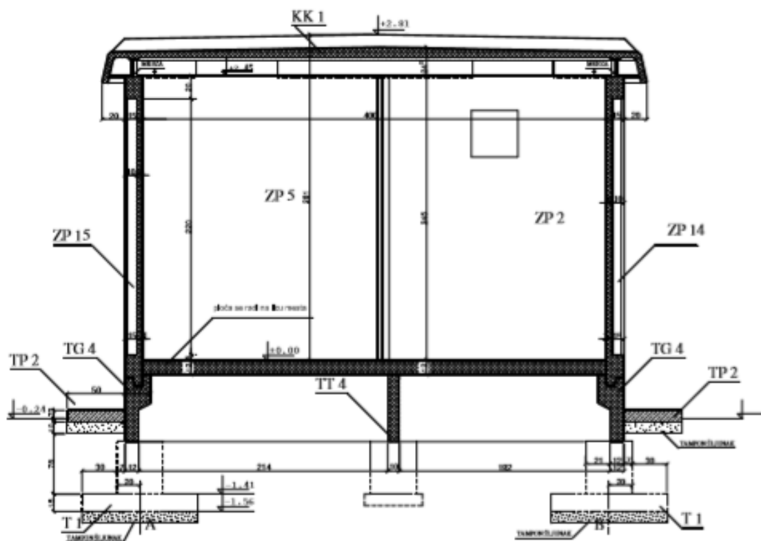
presek A - A, TP BP 19
